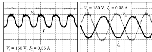
図6 入出力電圧電流観測波形 (a)入力側電圧電流 (b)出力側電圧電流 vd : 200V/div., I : 10A/div., va : 100V/div., ia : 10A/div.
